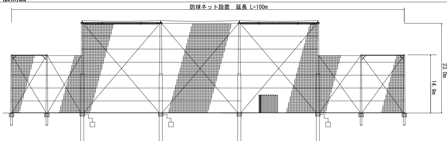
展開図
