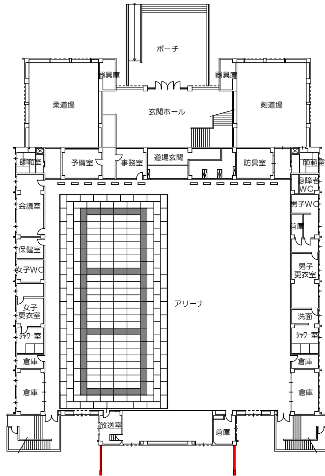
1階平面図 S = 1/500
