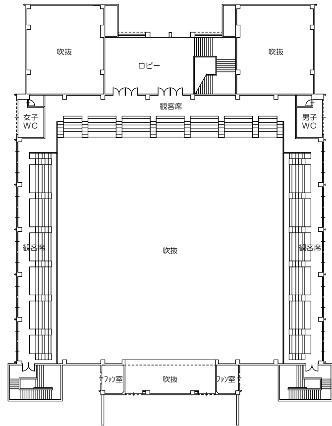
2階平面図 S = 1/500
