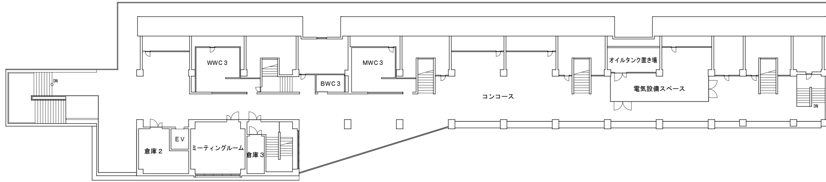
2階平面図
